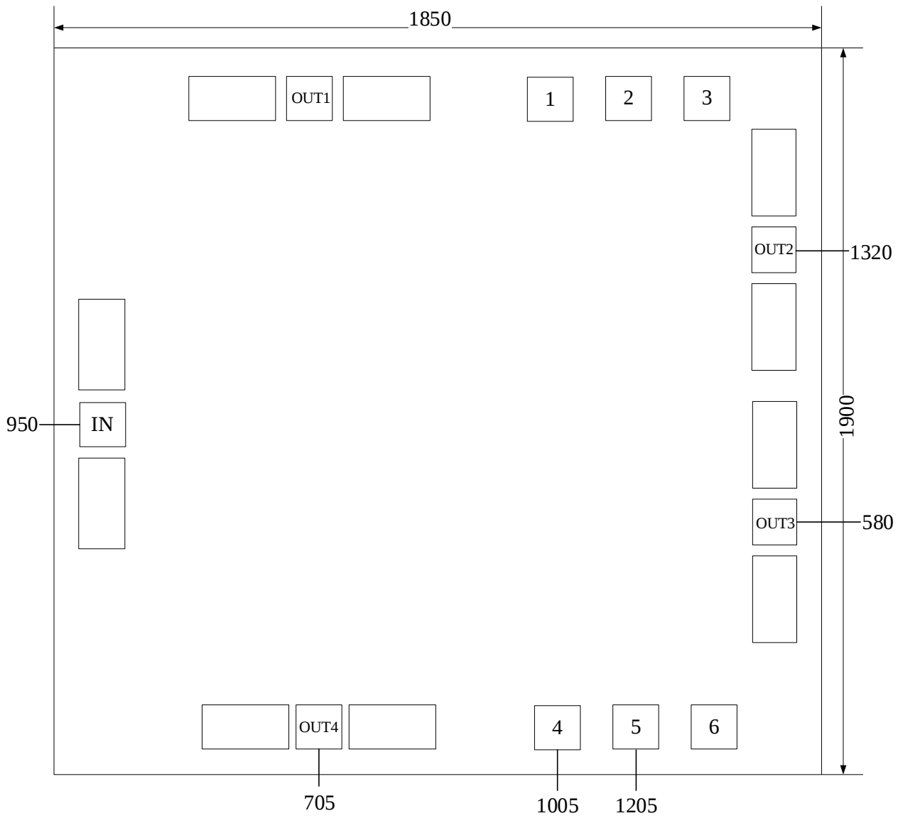
引脚定义
