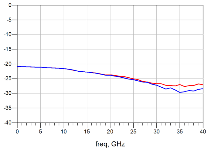
回波损耗
