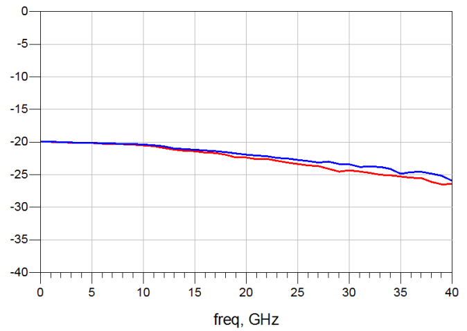
回波损耗
