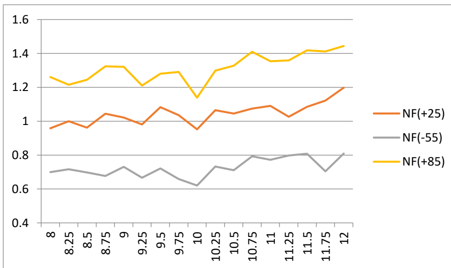
噪声系数
