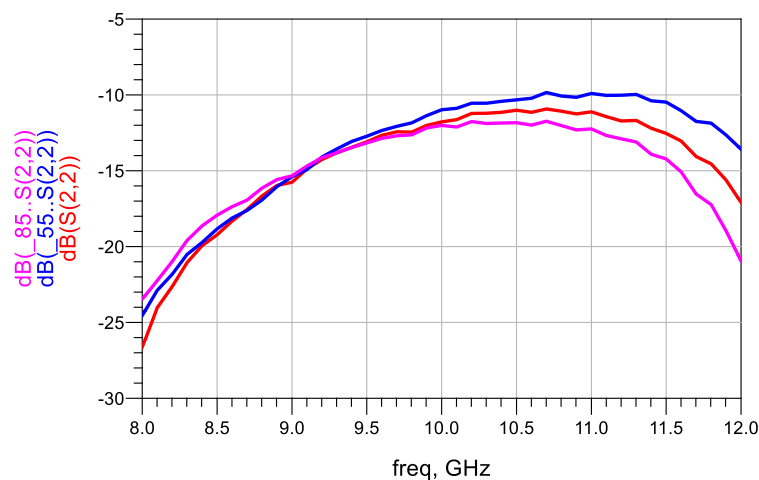
输出回波
