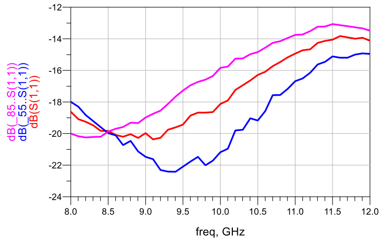
输入回波
