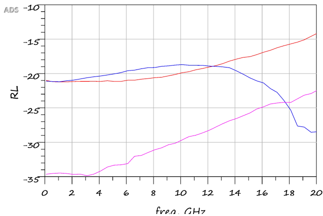
回波损耗
