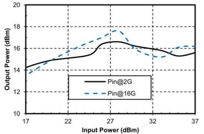
限幅电平 @2G & 16G
