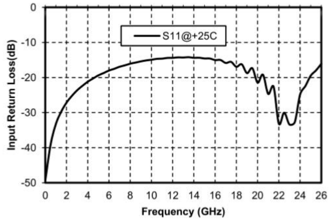
输入驻波 vs. 工作频率
