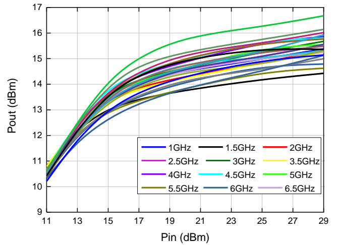
限幅电平
