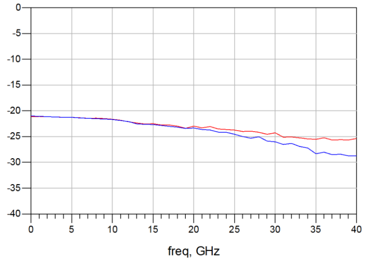
回波损耗
