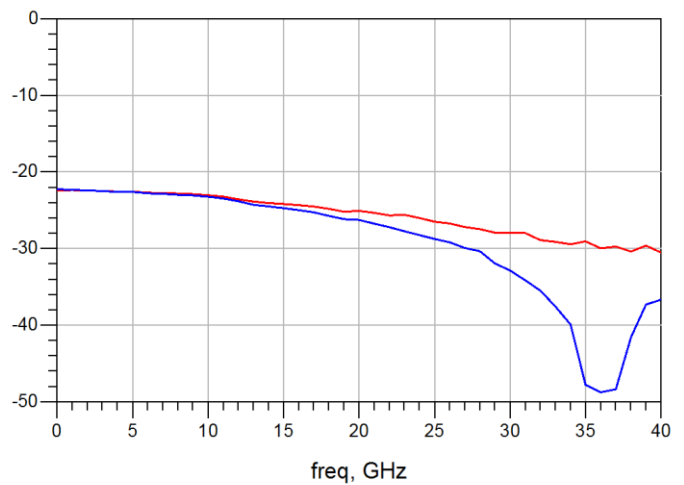
回波损耗
