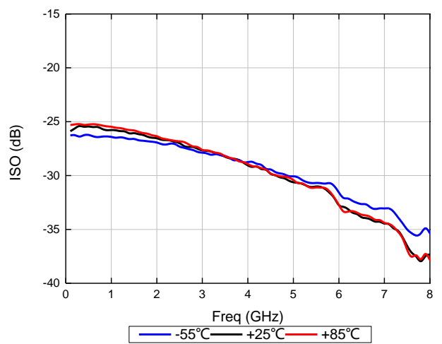
反向隔离度@低偏置
