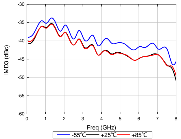
三阶互调@低偏置
