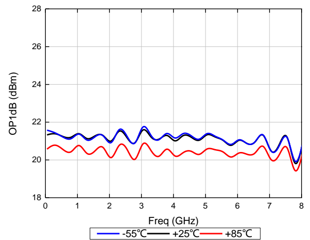
输出1dB压缩功率@低偏置
