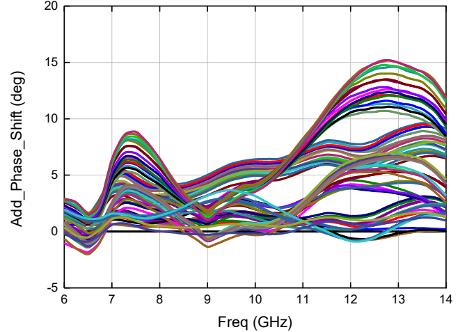
衰减附加相移
