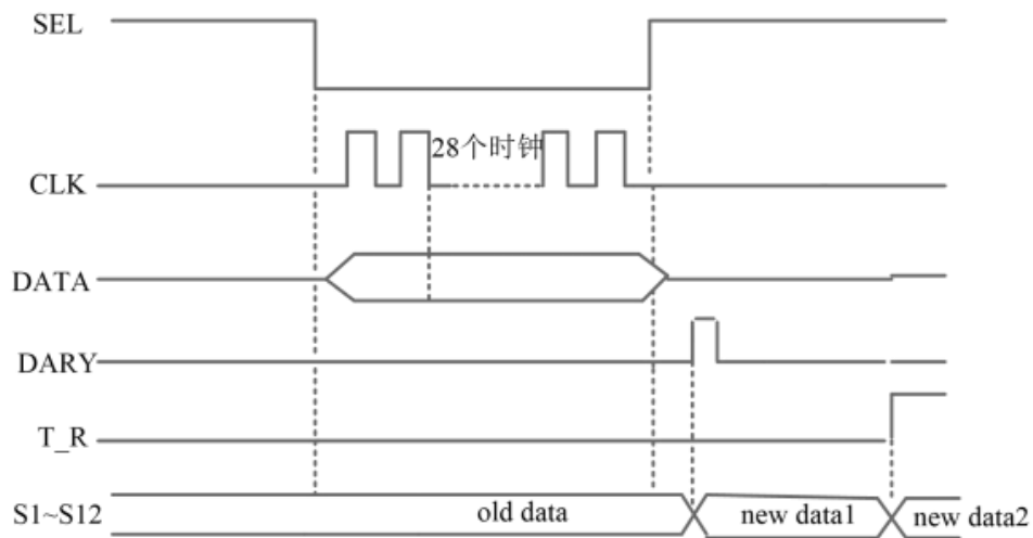
控制信号时序
