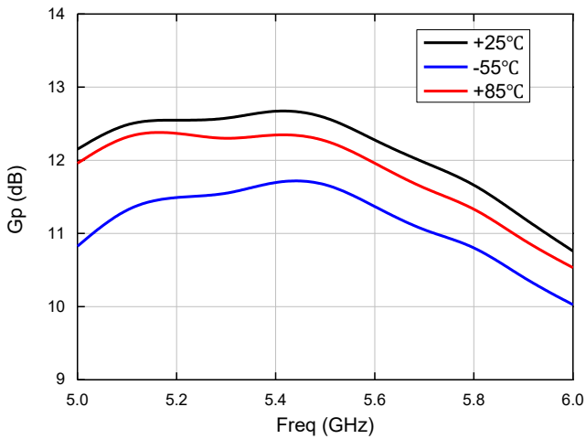
功率增益 (CW模式)
