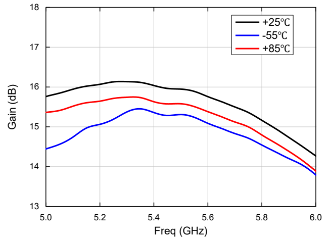
小信号增益
