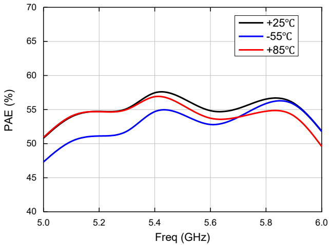
饱和功率附加效率 (CW模式)
