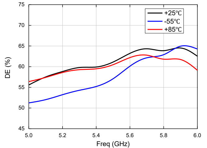
漏极效率 (Pulse模式)
