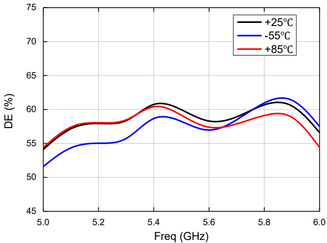
漏极效率 (CW模式)
