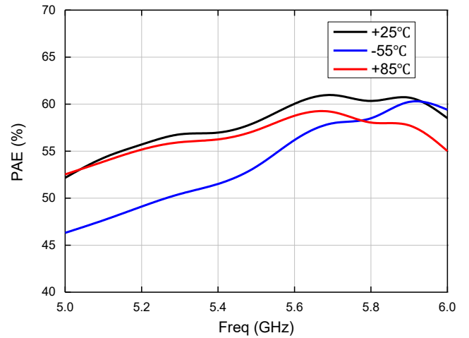
饱和功率附加效率 (Pulse模式)
