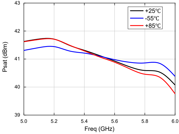
饱和输出功率 (CW模式)
