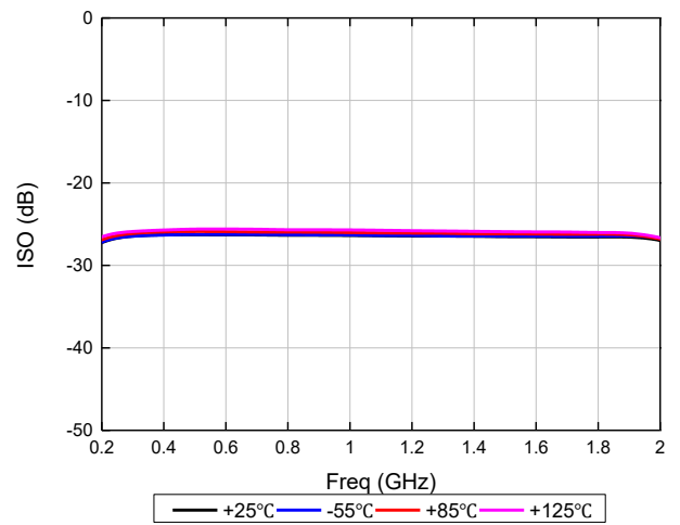
反向隔离度
