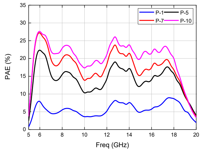
功率附加效率 (CW模式)
