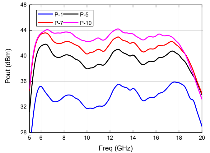
输出功率 (CW模式)
