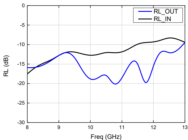
发射回波损耗 (Pulse)
