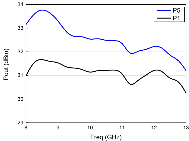
发射输出功率 (Pulse)
