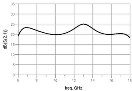
小信号增益 vs. 频率 (P in =-10dBm)
