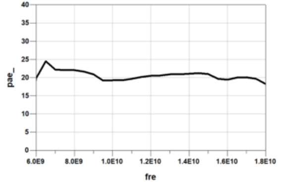
附加效率 vs. 频率 (P in =19dBm)
