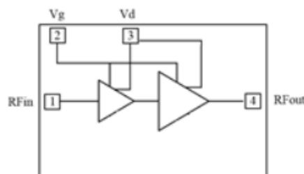
YGPA21-0618C1 功能框图
